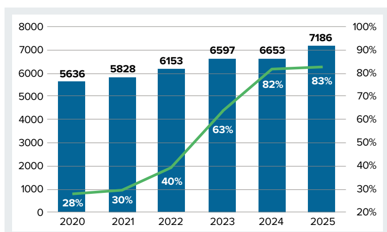
Viimsi valla teevalgustuse valgustite arvu muutus jaanuari alguse seisuga viimase kuue aasta lõikes, kõrvutatuna LED-valgustuse osakaalu kujutava kõveraga.
