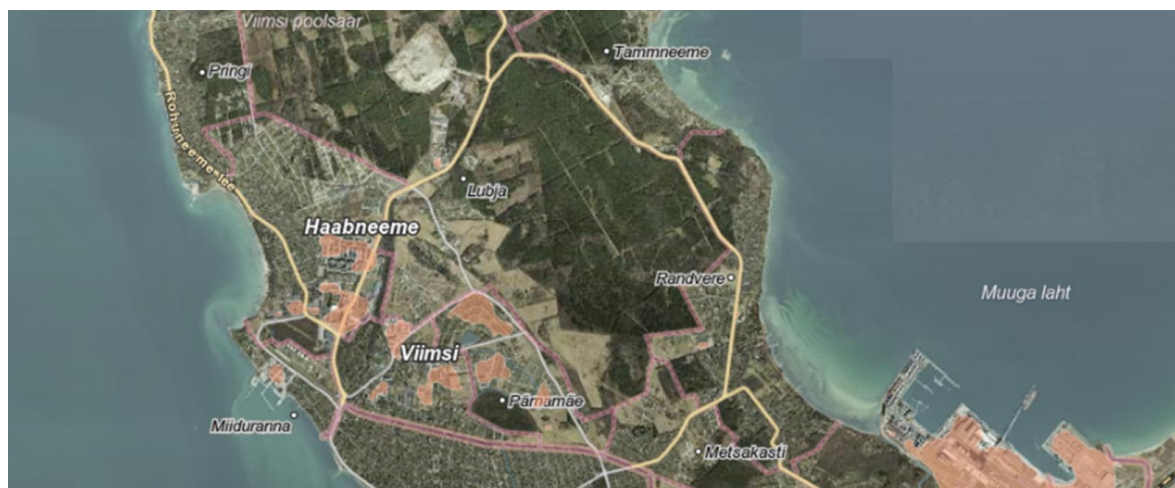
Joonis 16. Soojussaared Viimsi vallas 27. juulil 2014 (Maa-ameti geoportaal).
