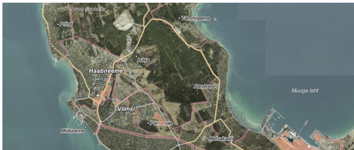
Joonis 17. Soojussaared Viimsi vallas 27. juulil 2018 (Maa-ameti geoportaal). Soojussaared arvatatud Landsat8 satelliitpildi pinnatemperatuuridelt kuumaperioodi alguses.
