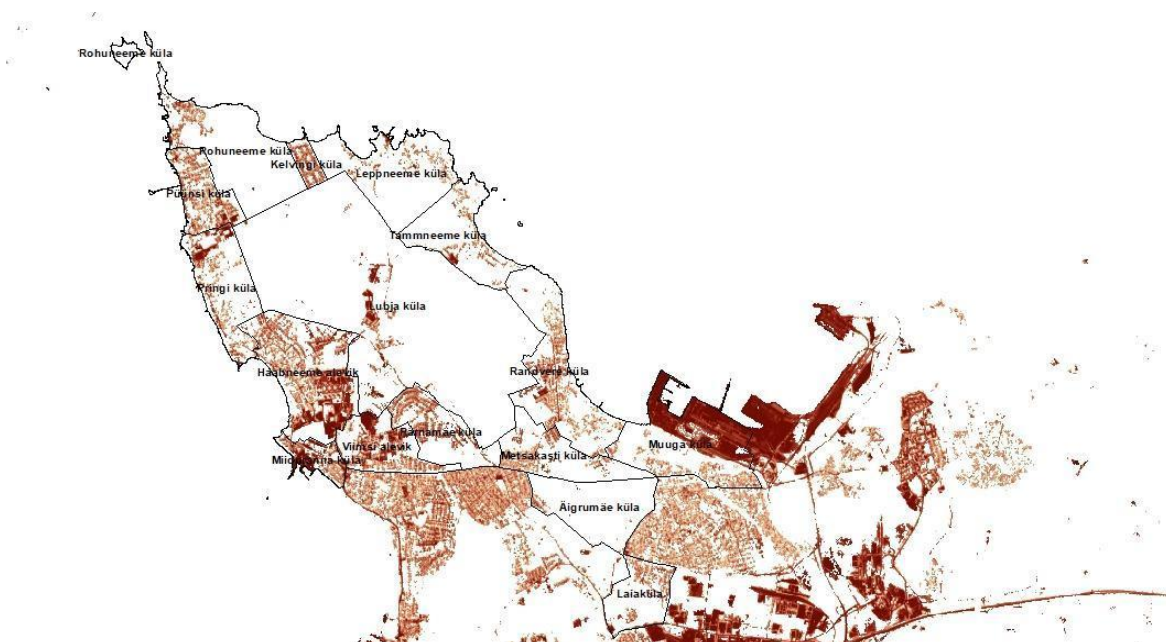
Joonis 1. Vett mitteläbilaskvate pindade (hooned, rajatised, teed jne) osakaal (0-100%) 10x10m rastris, Viimsi valla mandriosa 2018. aastal. Allikas: Copernicuse kaugseire portaal
