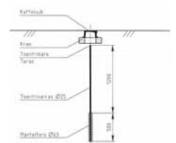
Paigaldatav märk tüüp 5030.
