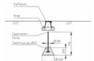
Paigaldatav märk tüüp 4623.
