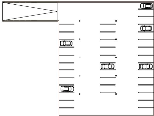
0. Korruse plaan
